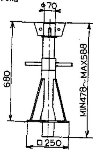
床ジャッキ YJ-40 W=31.5kg
