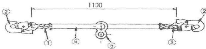
台付ロープ (TH-1型)
