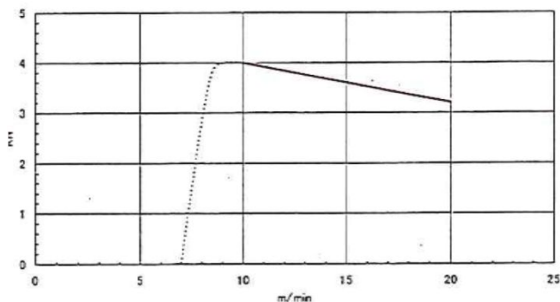
TPS-400E性能検図
