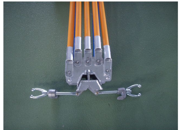
取付部詳細
