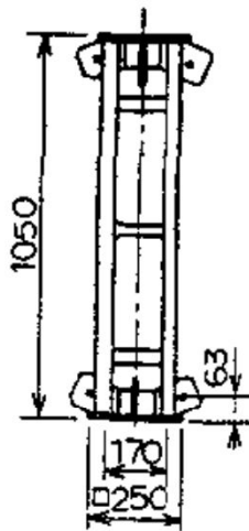
SE-105 W=30.2kg
