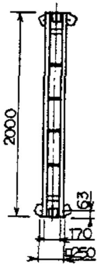
SE-200 W=42.1kg
