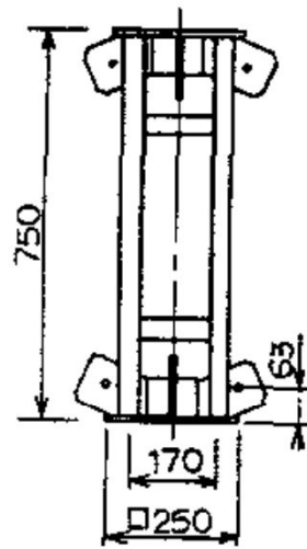
SE-75 W=26.3kg
