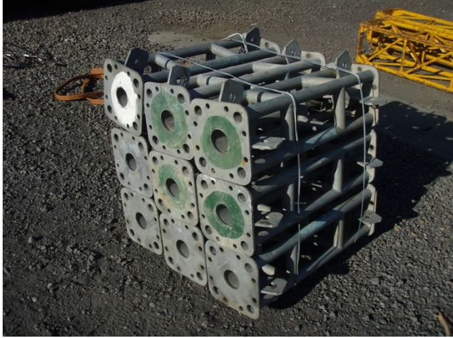
SE-105 W=30.2kg
